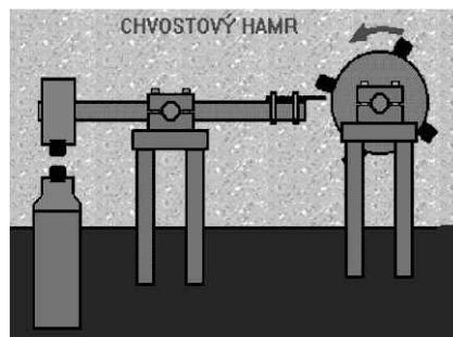
Schéma principu středověkého hamru
