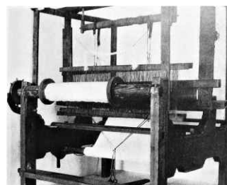
Tkalcovský stav
